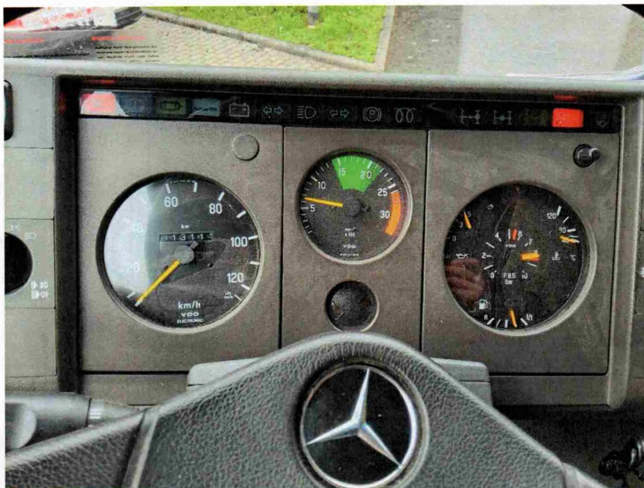
Bild 4 : Kombiinstrument
