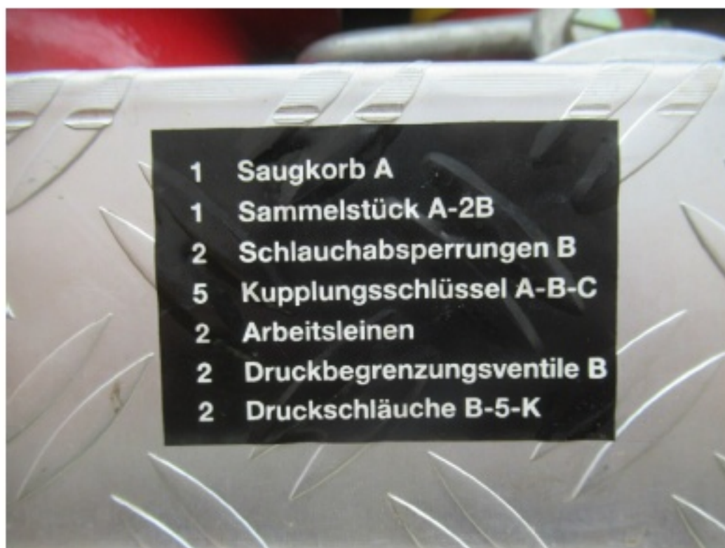
Bild 15 : Materialliste
