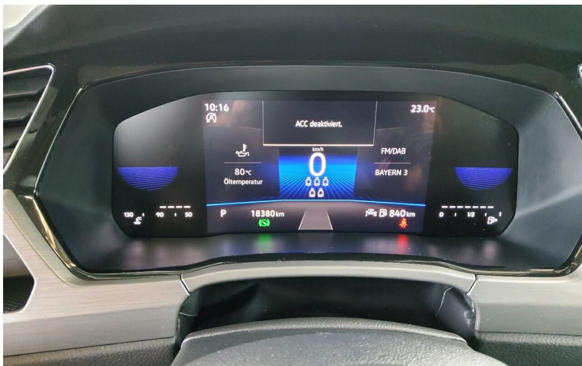
Bild 4 : Kombiinstrument
