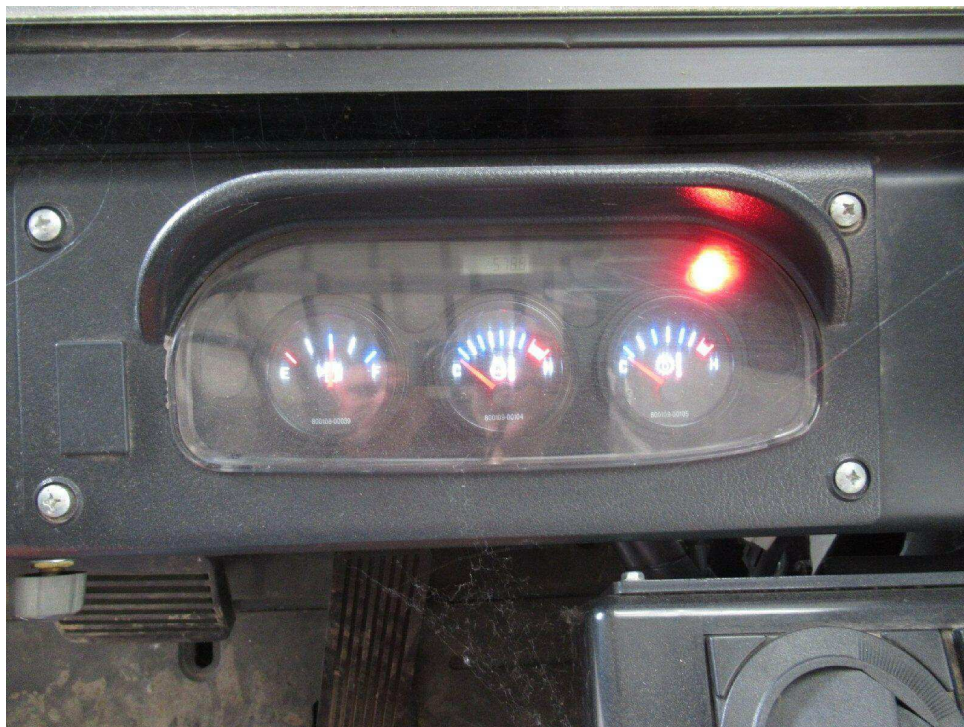
Bild 7 : Stundenzähler + Anzeigeeinstrumente
