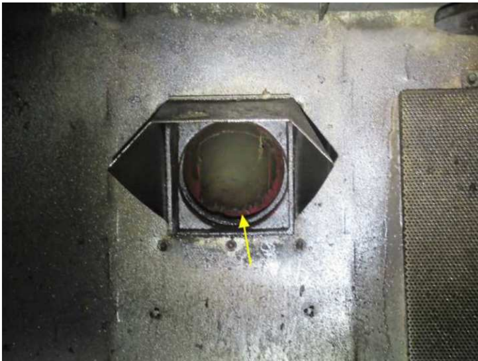
Bild 20 : Schiebevorrichtung für den Absaugkanal defekt
