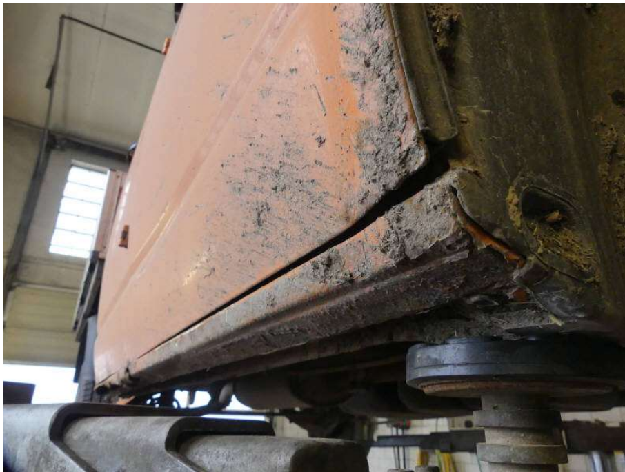
Bild 16 Unterholm rechts
